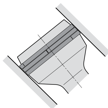
Поршень F3 с многослойным поршневым кольцом.
