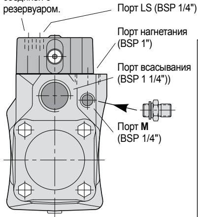
Вид торца VP1-45/75 (показаны порты).
