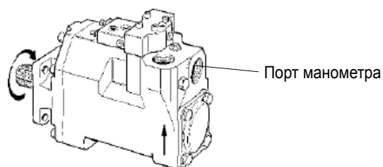
Рис. 4. Насос с направлением вращения против часовой стрелки.
