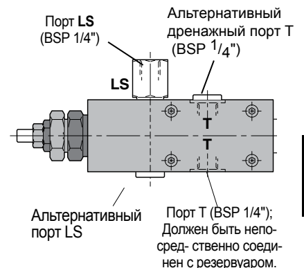
Порты регулирующего клапана VP1-095/-110/130.
