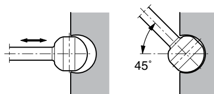
Соединение поршня и вала F3.
