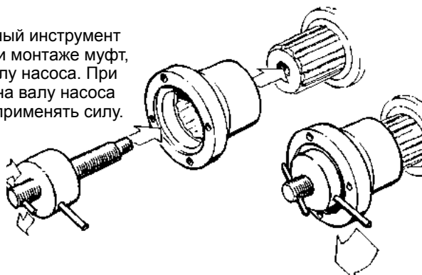
Рис. 7. Монтажный инструмент.
