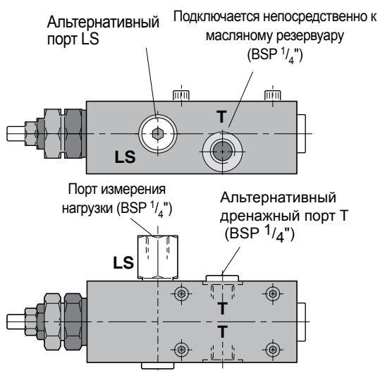
Порты регулятора с измерением нагрузки.
