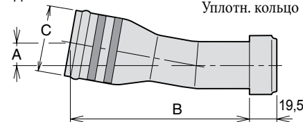
Соединение 45°
