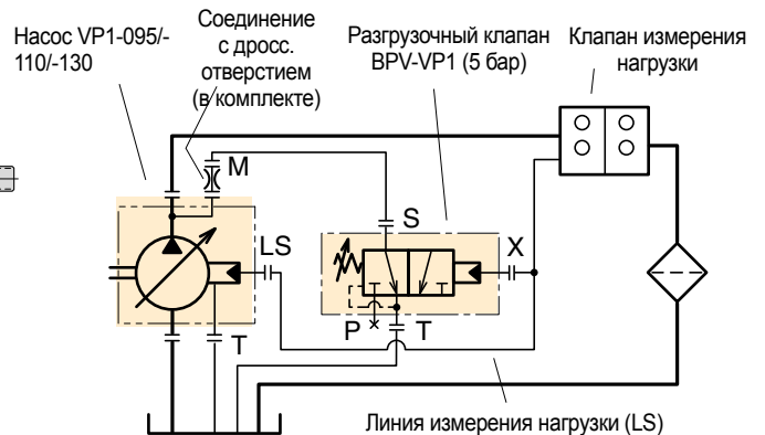
Схема монтажа клапана BPV-VP1 с насосом VP1-095/-110/-130
