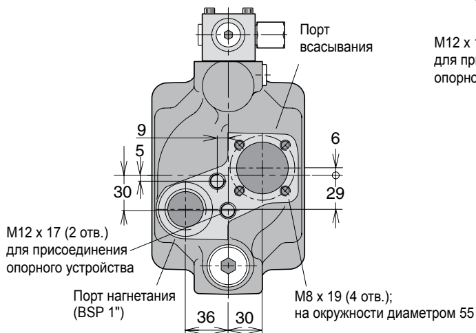
Вид А-А насос с вращением против часовой стрелки
