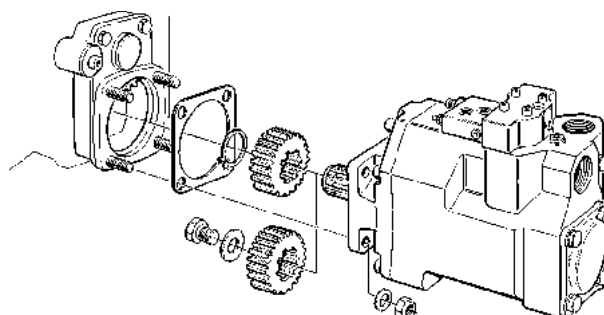
Рис. 6. Монтаж VP1 на коробке отбора мощности.
