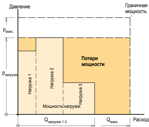
Диаграмма 1. Система с постоянным расходом с нерегулируемым насосом.
