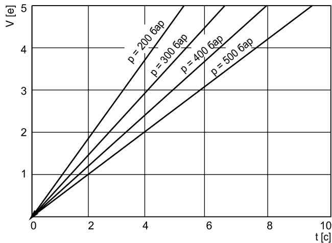
Все характеристические кривые измерены с использованием масла HLP46 при 50°C.
