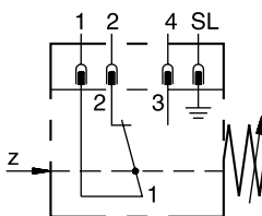
Электрическое соединение согласно EN175301-803
