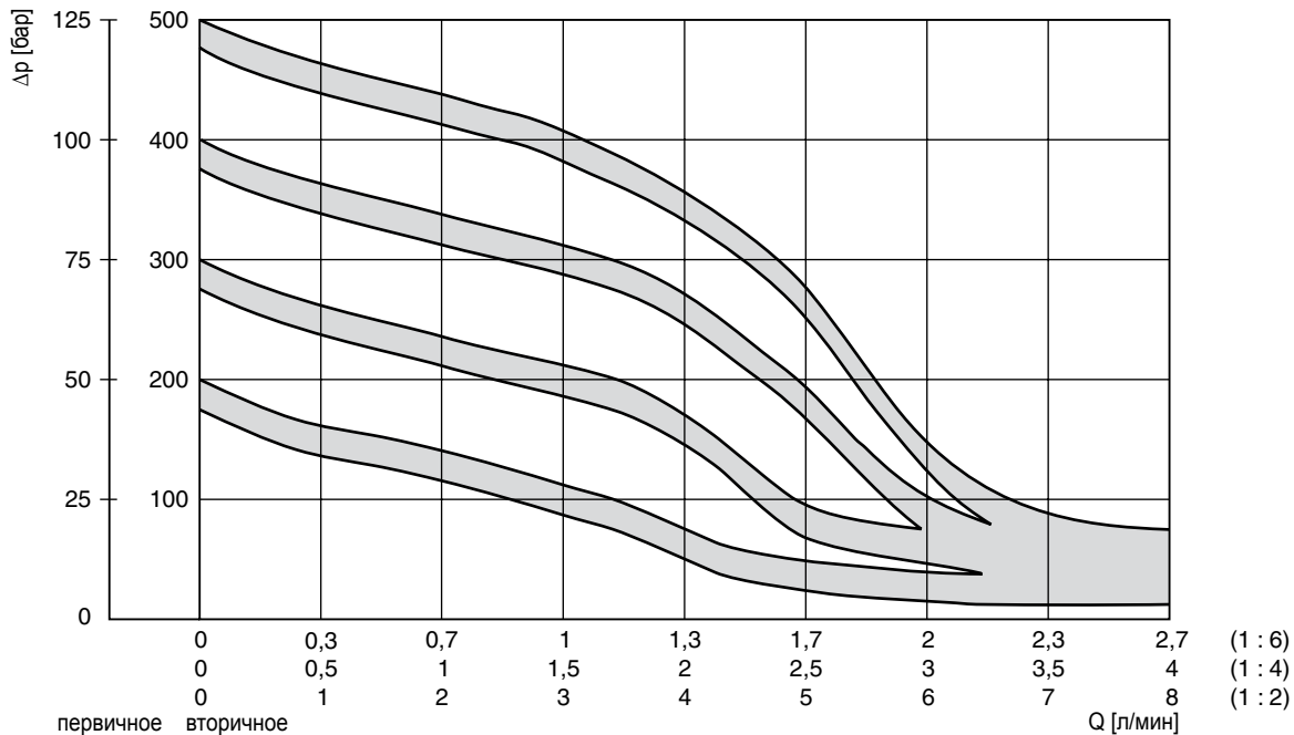
Примерные значения времени сжатия жидкости в заполненной секции до заданного давления (1 : 4)
