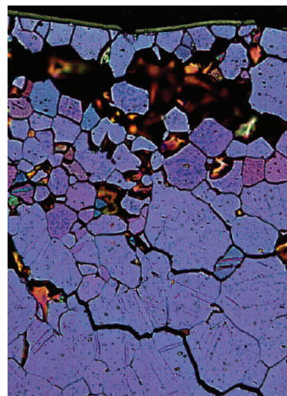
Коррозионное растрескивание нержавеющей стали под нагрузкой в морской воде
