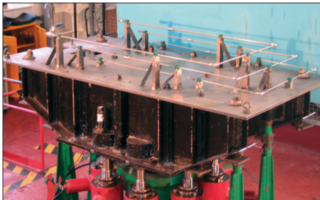
Испытание на ударную прочность
