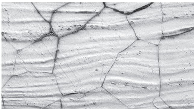
Межкристаллитная коррозия – Зона теплового воздействия (HAZ) – Сварной шов из нержавеющей стали в морской воде
