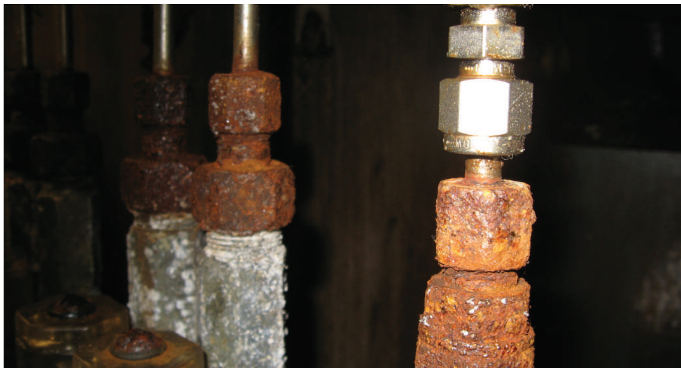
Электрохимическая реакция, создаваемая смешиванием разных материалов для корпуса и гайки.
