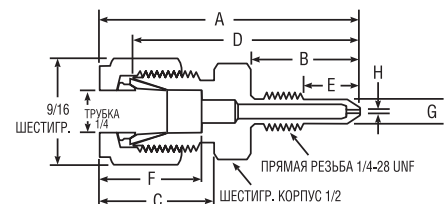
Переходник для калибровки датчиков перепада давления Honeywell
