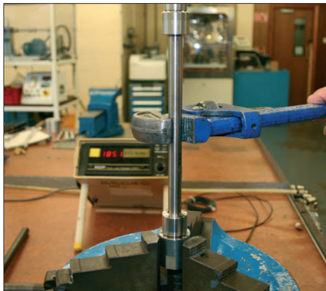
Испытание вращением
