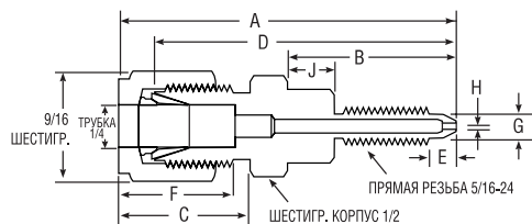
Переходник для калибровки датчиков перепада давления Rosemount/Foxboro
