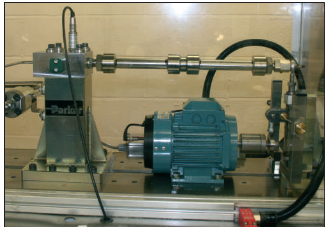
Вибрационное испытание
